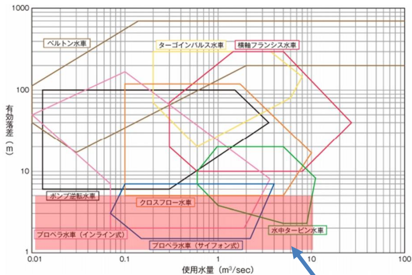
推奨作動領域 Recommended operating area of 【WaterWeco®】
