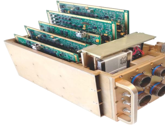
1553B & FIM Card
